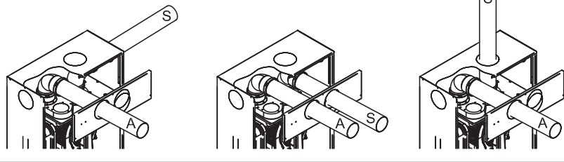
Esempi di sistemi con aspirazione diretta B_{23}
